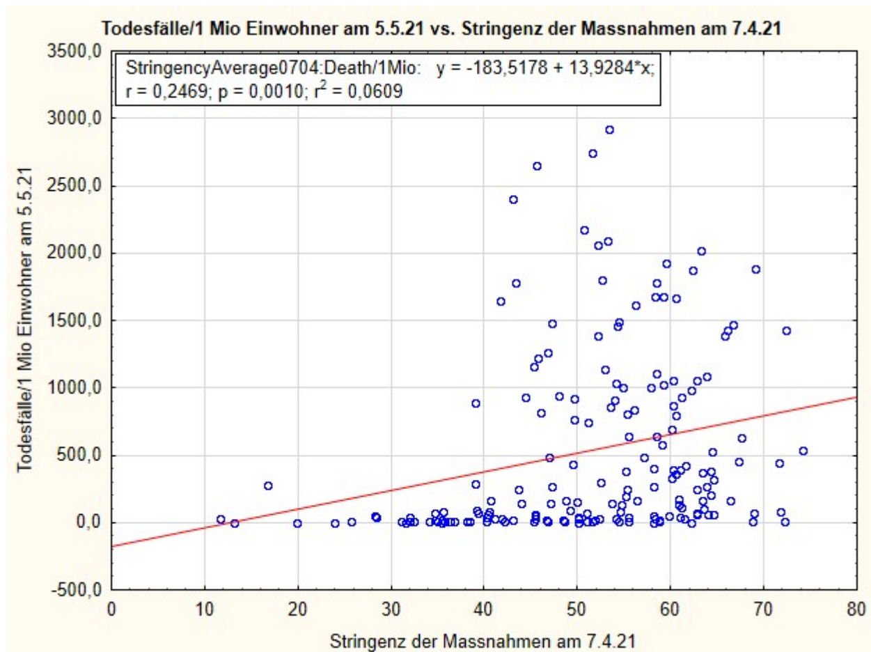
Abbildung 2 – Zeitversetzte Korrelation der Stringenz der Maßnahmen vor einem Monat (7.4.21) mit den Todesfällen heute (5.5.21) (Daten: https://www.worldometers.info/coronavirus/ vom 5.5.21 und Oxford Policy Tracker am 7.4.21)
