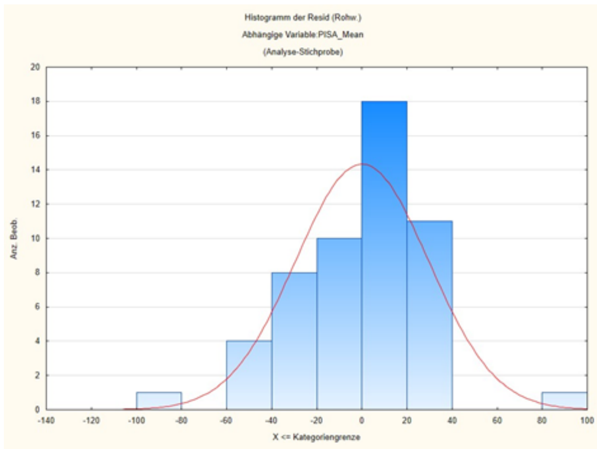
Abb. 2 - Histogramm der Residuen
