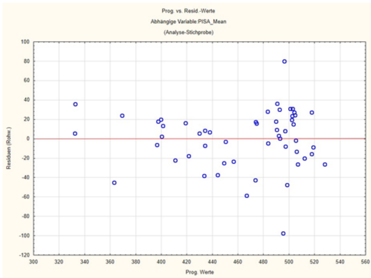
Abb. 3 – Plot der Residuen vs. vorhergesagte Werte
