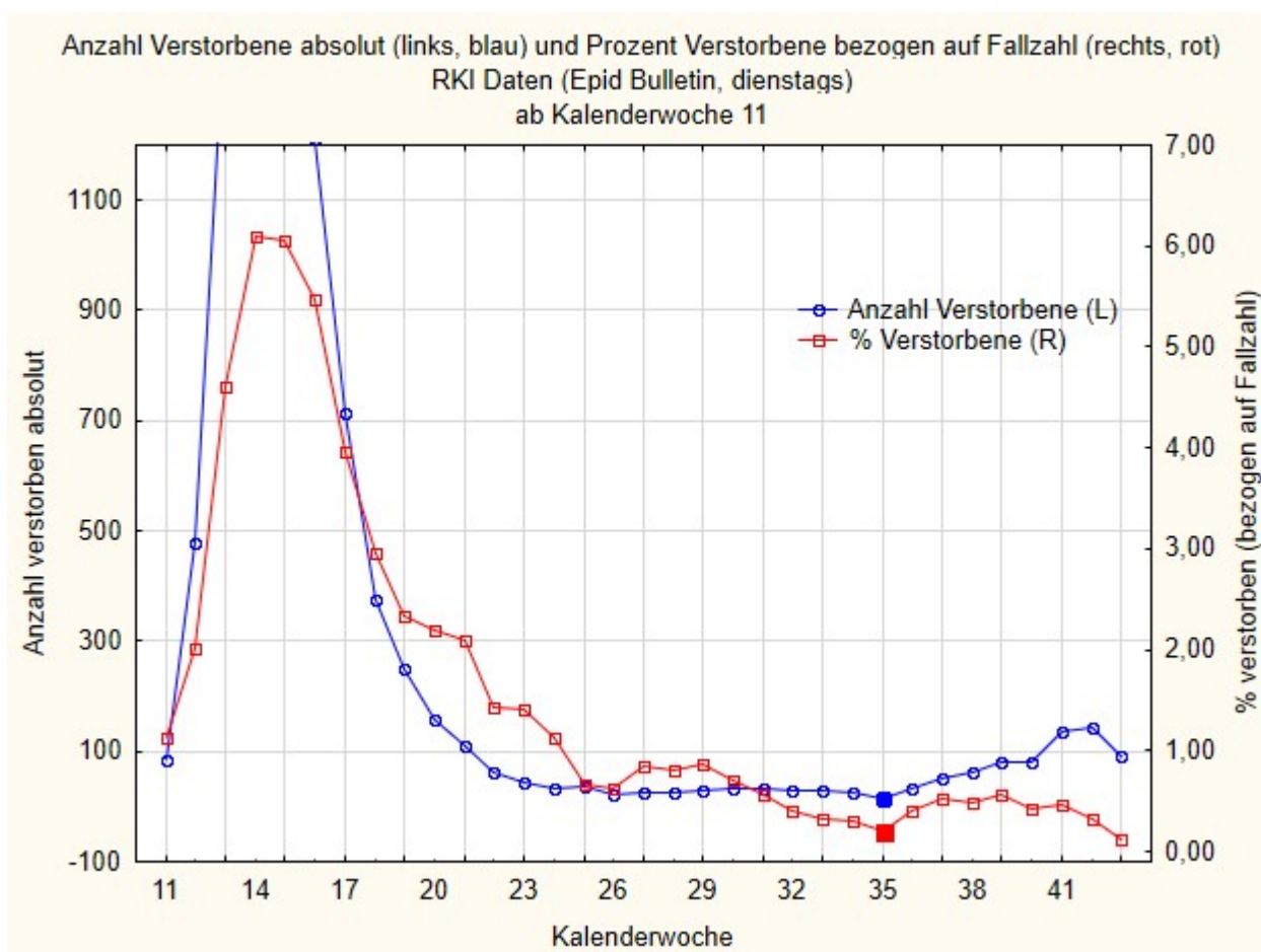
Abbildung 3 - Anzahl der Verstorbenen, deren Tod mit SARS-CoV2 in Verbindung gebracht wird (Daten RKI Wochenberichte vom 28.10.20); blaue Kurve (linke y-Achse): Absolute Anzahl je Kalenderwoche ab 11. Kalenderwoche bis KW 43; rote Kurve (rechte y-Achse) prozentualer Anteil aller positiv Getesteten
